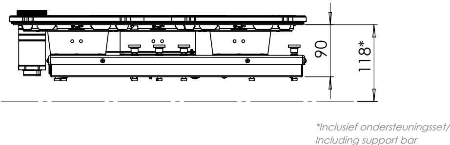
Zijaanzicht / Side view
