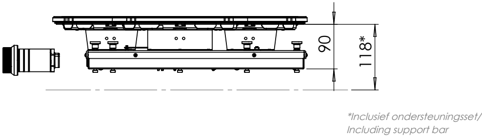
Zijaanzicht / Side view
