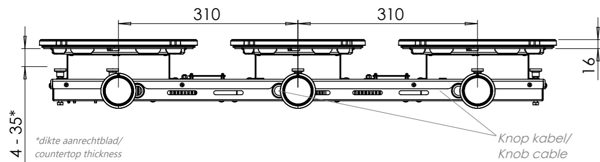
Vooranzicht / Front view
